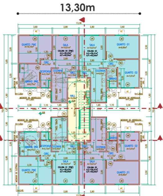
PLANTA BAIXA TÉRREO PNE (BLOCOS 1, 2, 5)
