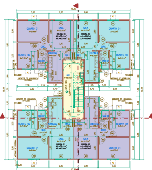
PLANTA BAIXA TÉRREO (BLOCOS 12, 13 e 22)
