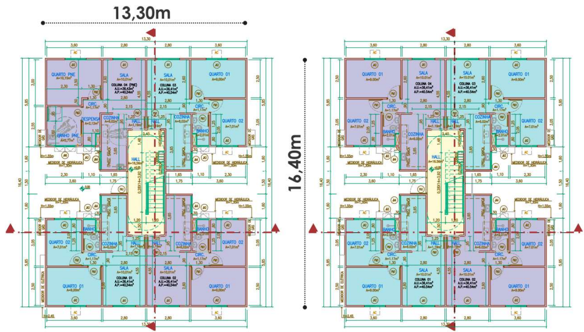
PLANTA BAIXA TÉRREO PNE (BLOCO 1)
