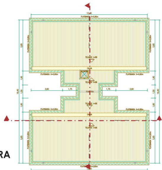
PLANTA BAIXA TÉRREO (BLOCO 18)
