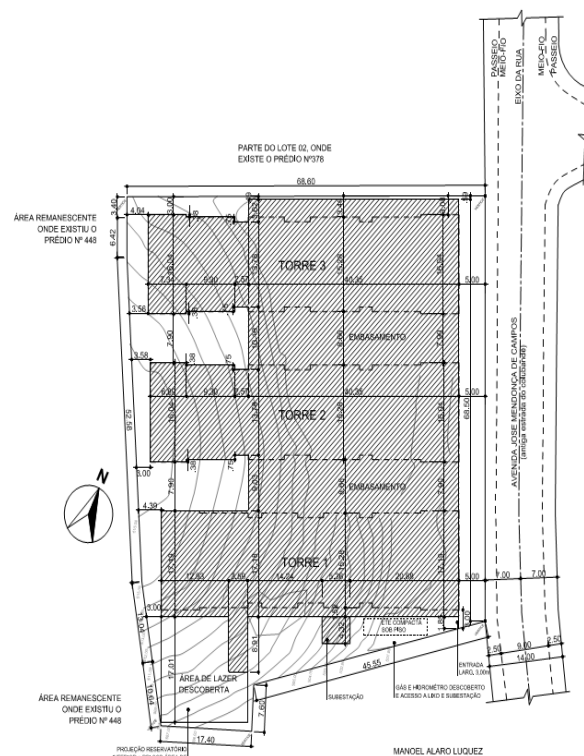
01 PLANTA DE SITUAÇÃO ESCALA 1:500
